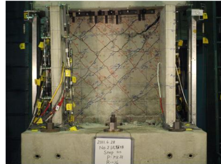
図 5 直交壁の耐震性検証実験
