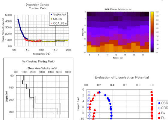
図 4 微動探査法の利用
